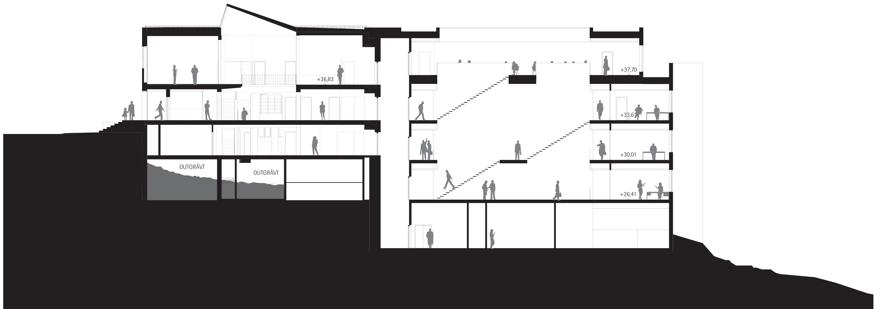
TVÄRSEKTION GENOM BEFINTLIGT HUS & TILLBYGGNAD
